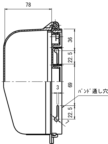
A-A断面図
