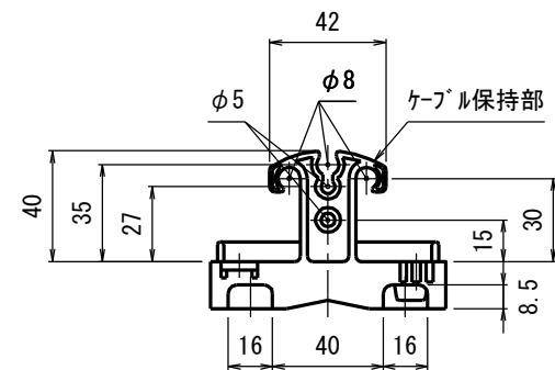
基台底面図
