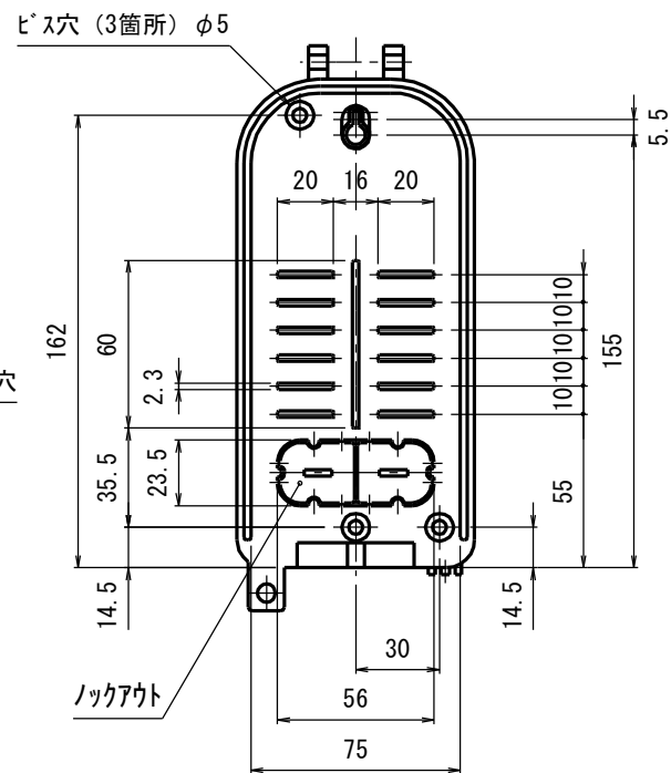
基台正面図
